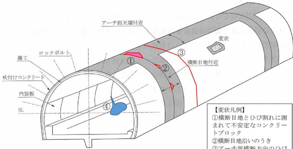
本トンネルに見られる変状種類と位置の模式図 「道路トンネル維持管理便覧【本工編】」平成27年6月 (公社)日本道路協会 P146の図に追記
